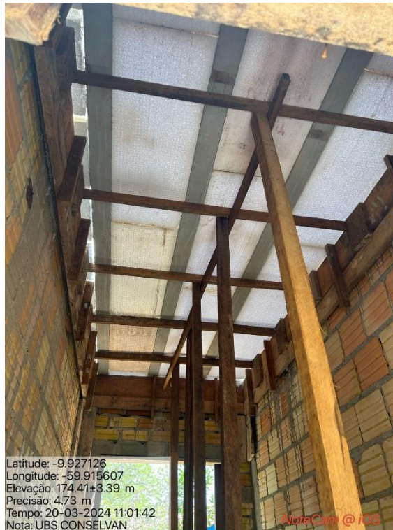
Escoramento de laje
